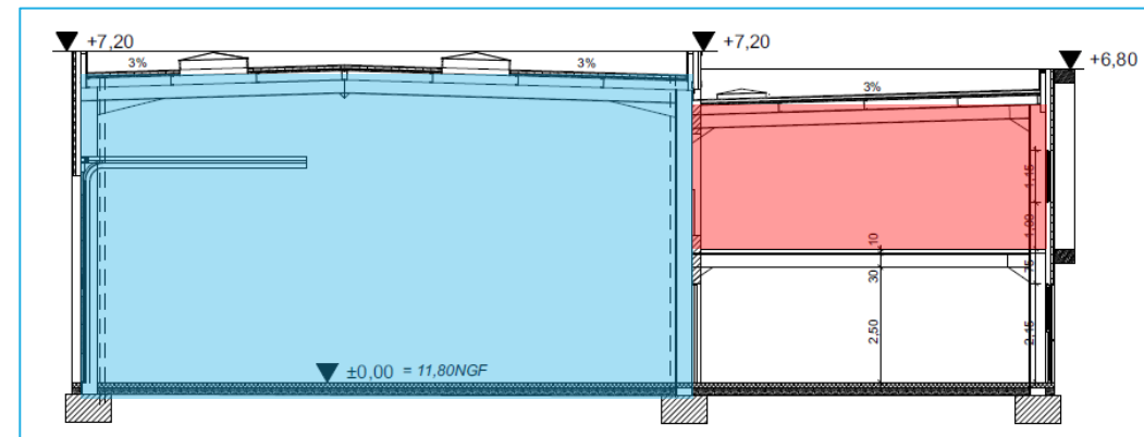
COUPE
