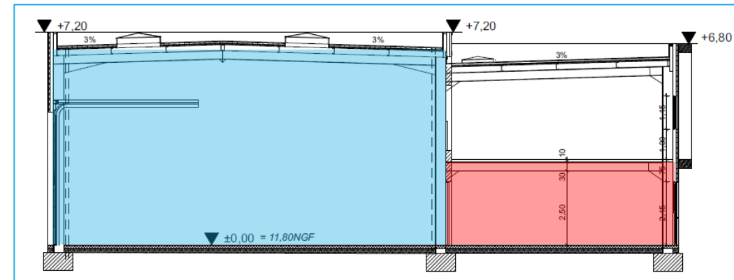
COUPE
